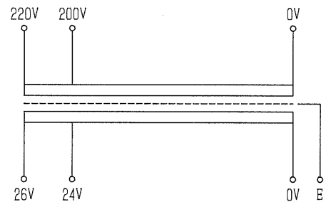
結線図
