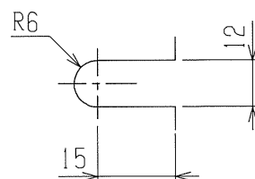
固定用穴詳細図
